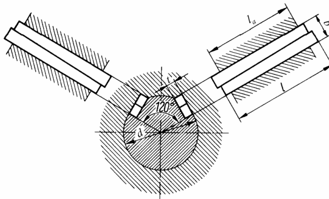
Sl. 16. Spoj tangentnim klinom
